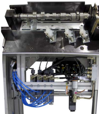
4 mazané miesta vačkového hradela
