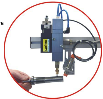
Celoživotné mazanie ložísk vretena pletacieho stroja
