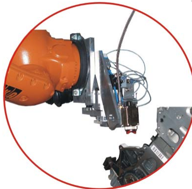
Nástrek silikónu na výrobné číslo bloku motora
