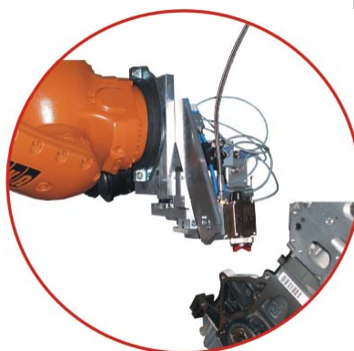
Nástřik silikonu na výrobní číslo bloku motoru
