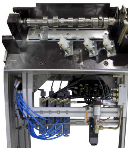
4 mazaná místa vačkové hřídele
